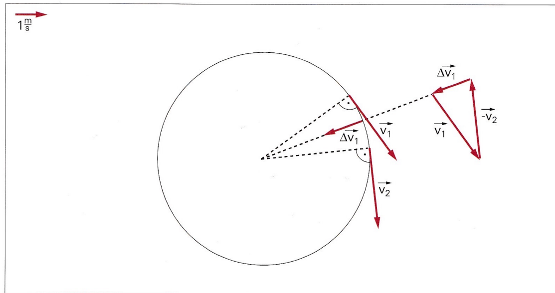
[Abb. 9.4] Vektoren der Geschwindigkeitsänderung
