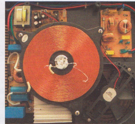
Figur 104 Induktionskochfeld: Spule
