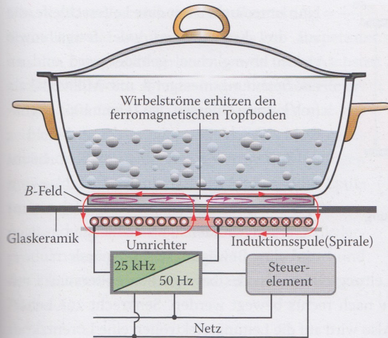
Figur 103 Induktionsherd: Prinzipschema
